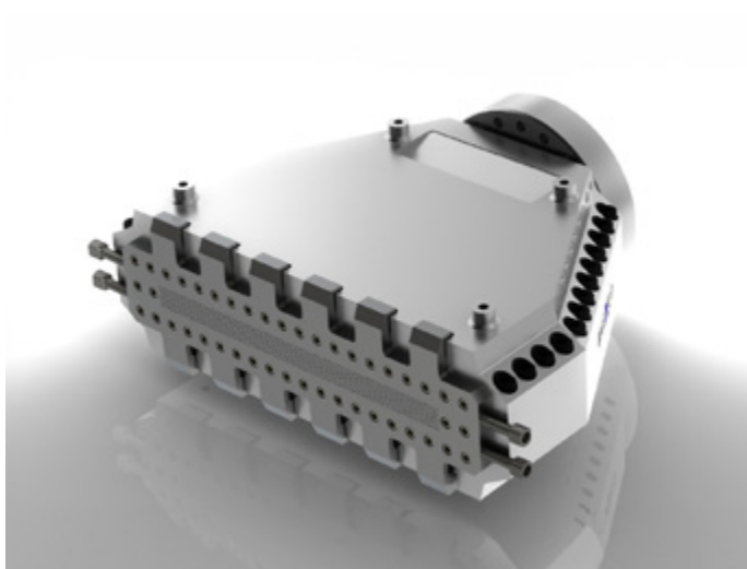
PET- FOAM SHEET EXTRUSION DIE
