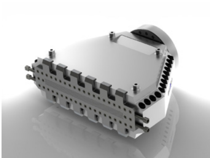
PET-PLATTENKOPF
